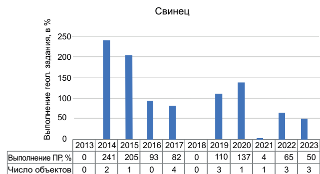
Рис. 3. Результативность ГРП (в %) по объектам Госзаказа по соотношению полученного и ожидавшегося по Госконтрактам прироста прогнозных ресурсов цветных и благородных металлов (кат. P_1 + 0,6P_2 , по [1]) в период 2013–2023 гг.
