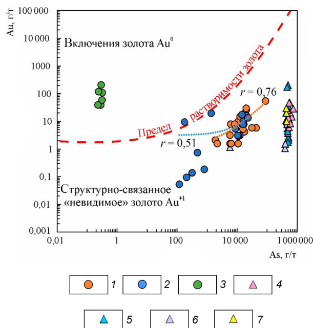
Рис. 5. Диаграмма концентраций Au-As в пирите и арсенопирите рудного поля Упрямое, по [35]:
