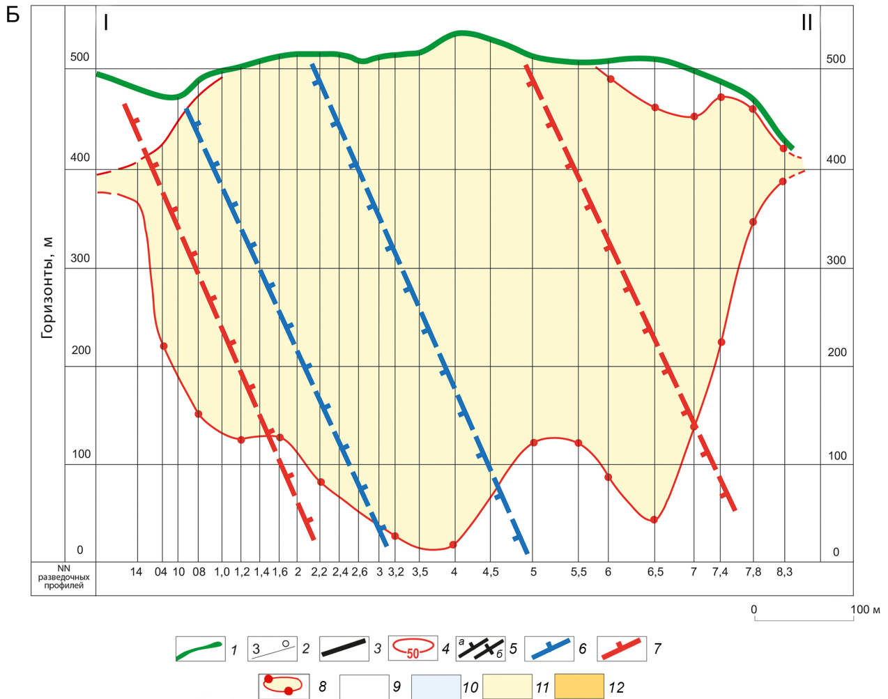
Рис. 28. Проекция на горизонтальную плоскость изолиний значений метрограммов в рудной зоне участка Ольга по скважинам и каналам (А) и проекция на вертикальную плоскость (линия I-II) контура балансовых запасов на рудной зоне участка Ольга (Б):
