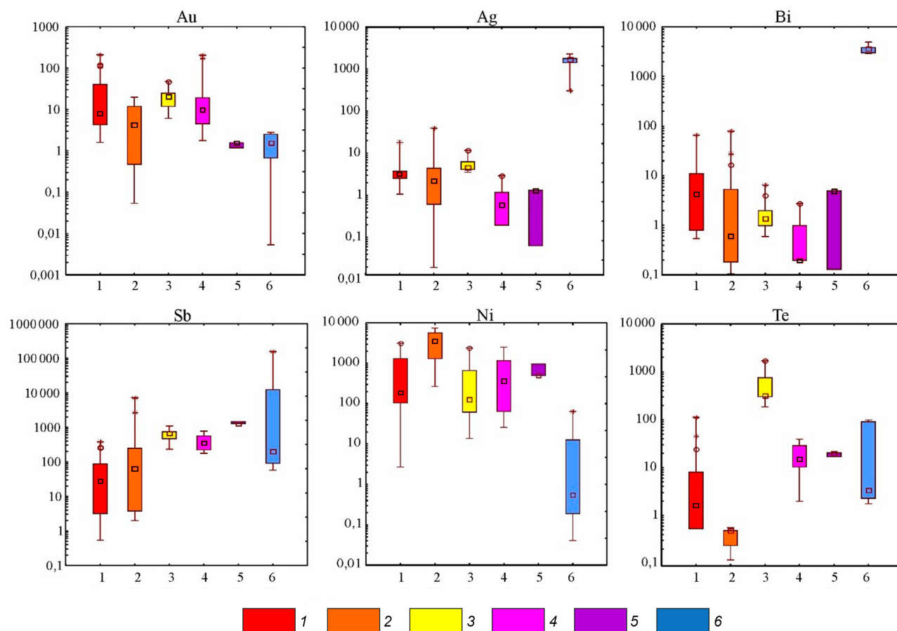
Рис. 3. Диаграммы размаха содержаний элементов-примесей в главных рудных минералах рудного поля Упрямое:
