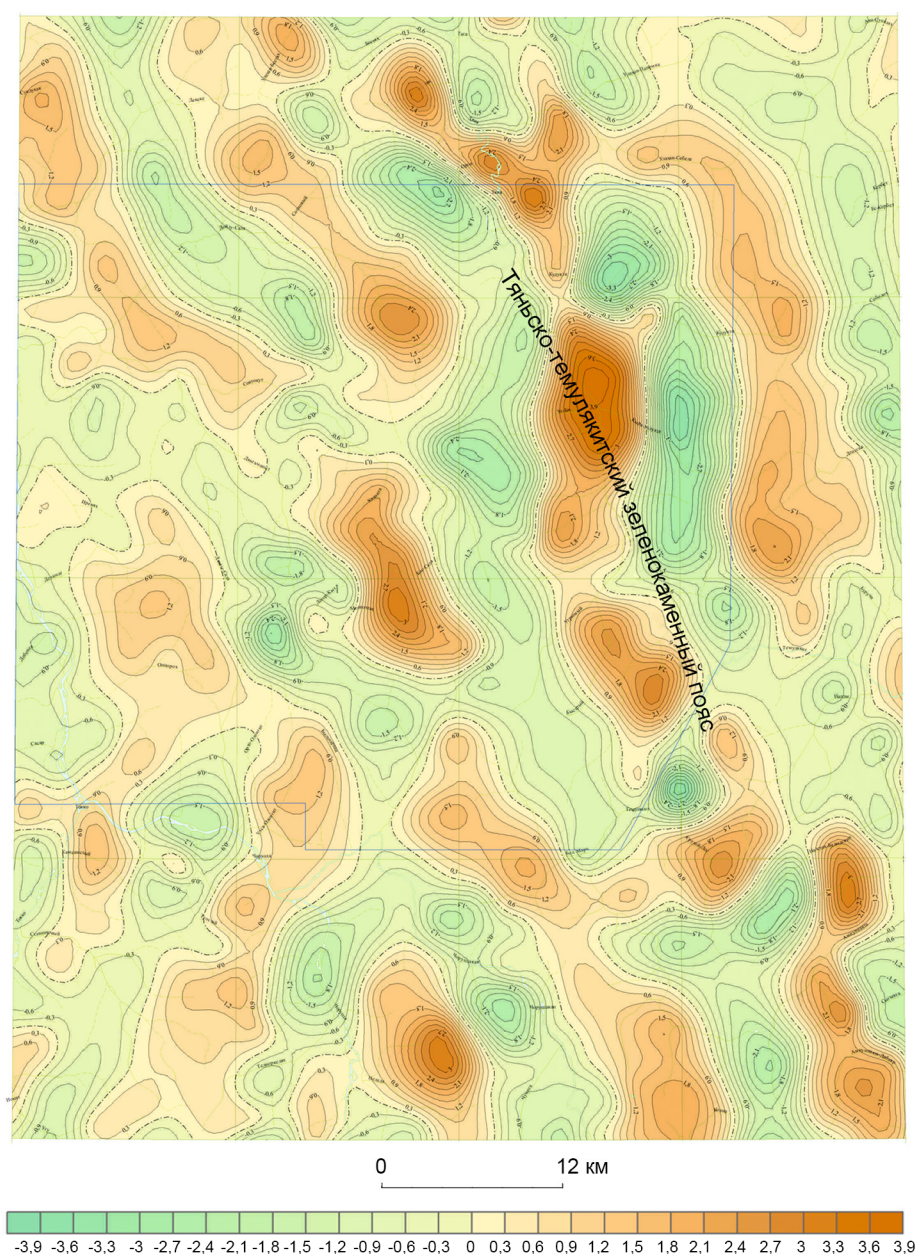
Рис. 2. Проявленность Тяньско-Темулякитского зеленокаменного пояса на карте изолиний локальной составляющей поля силы тяжести. Значения поля приведены в условных единицах
