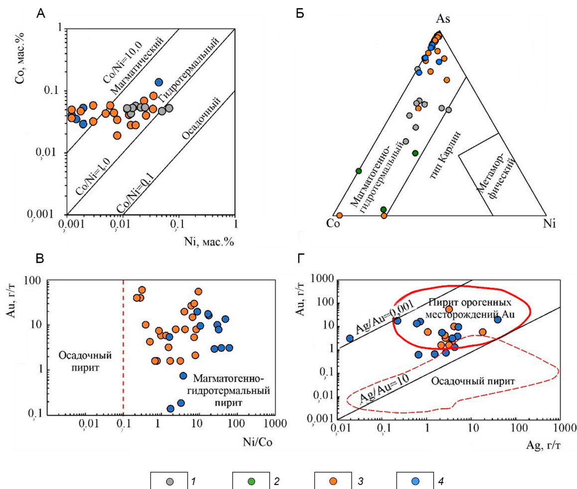
Рис. 6. Диаграммы состава пирита: А – Co–Ni, по [18], Б – As–Co–Ni, по [38], В – Au–Ni/Co, по [32], Г – Au–Ag, по [25]:
